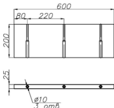
Дюбель фасадный под ключ 10x200
